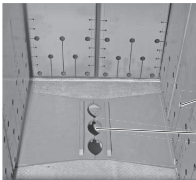
Fig. 43 Füllraum, Löcher in Einhängbleche, Durchbrandöffnung
